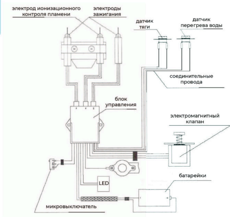
Рис.2. Схема электрическая
