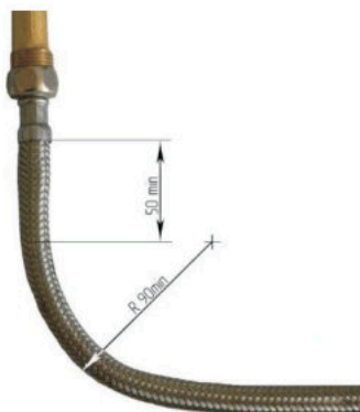
Рис. 2. Требования к монтажу гибких шлангов
