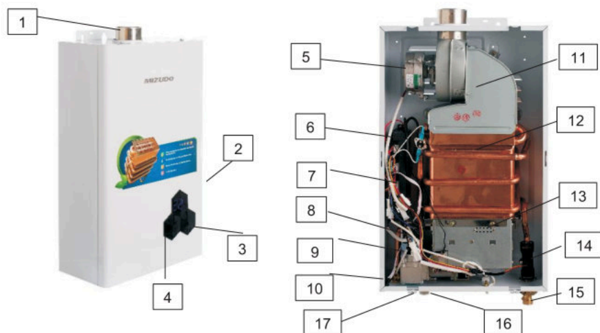
Рис. 1. Аппарат водонагревательный проточный газовый бытовой
