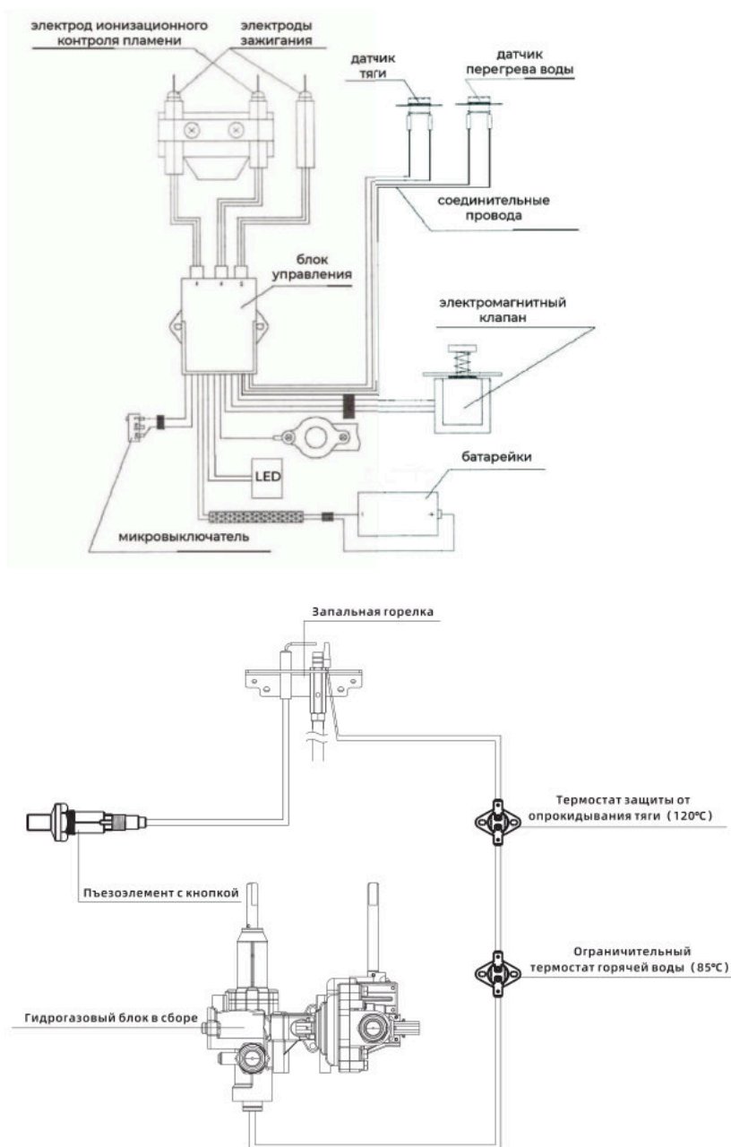
Рис.2. Схема электрическая
